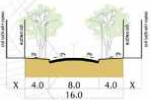
CẮT 3-3
