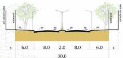
CẮT 1-1
