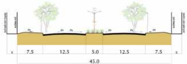
CẮT 1A-1A
