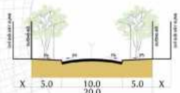
CẮT 2-2
